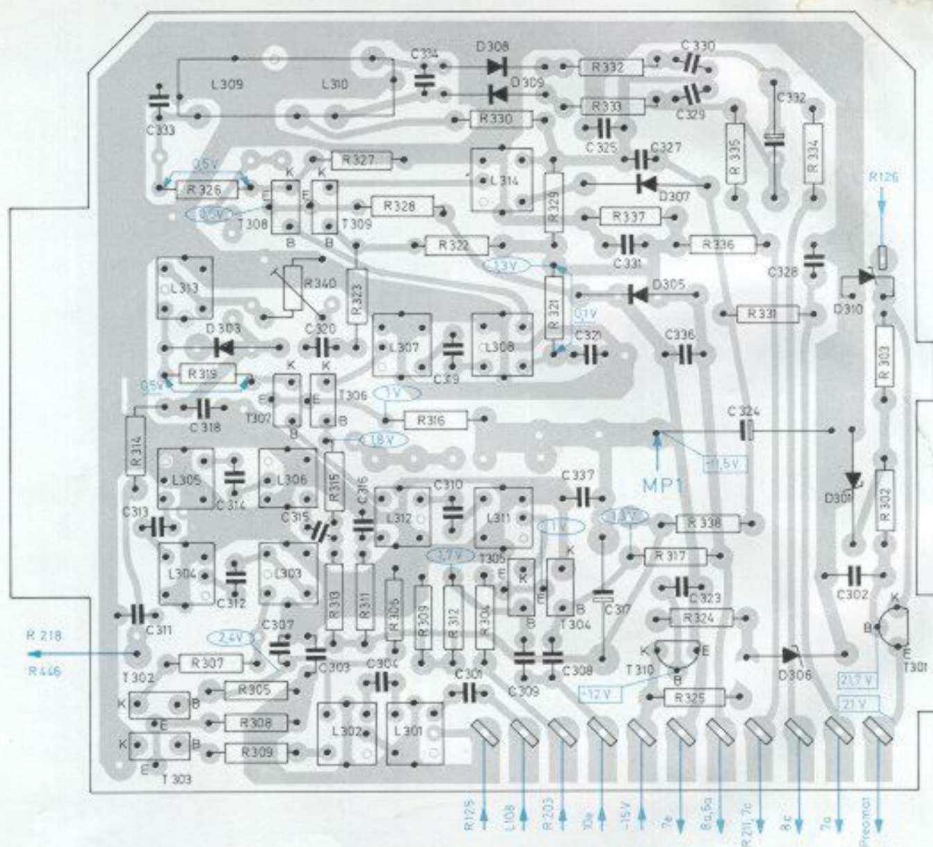
Fig. 4 ZF-Teil 231 220 (Leiterseite)
