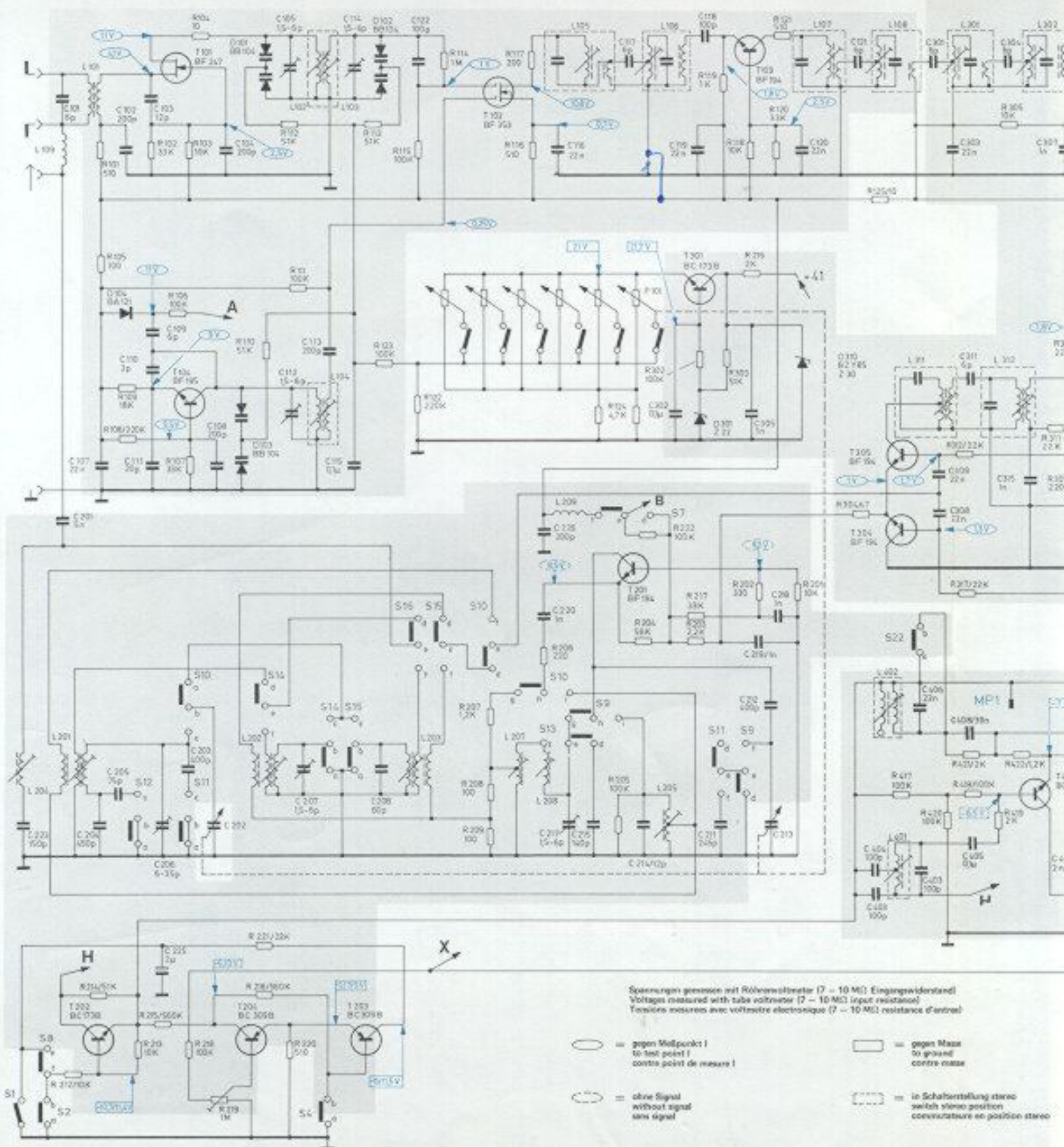
Fig. 3 Schaltbild HF
